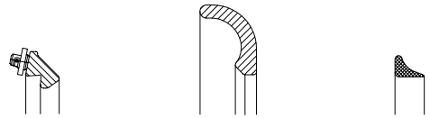
LOCK RING Kilit Halkası (Segman)
