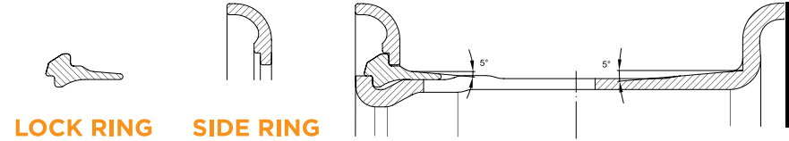
LOCK RING Kilit Halkası (Segman)
