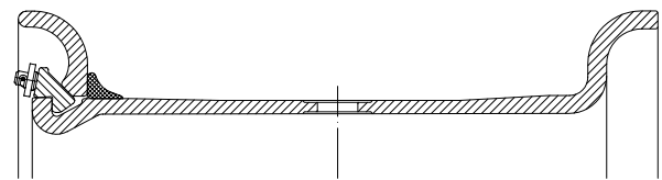
LOCK RING Kilit Halkası (Segman)
