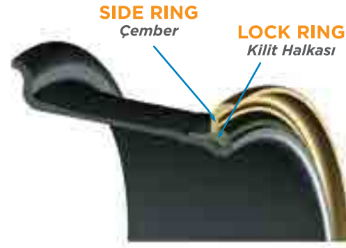
3 PIECE TYPE 3 Parçalı Model
